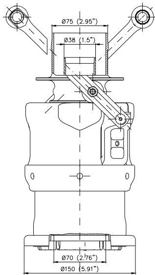
Accoupleur femelle
