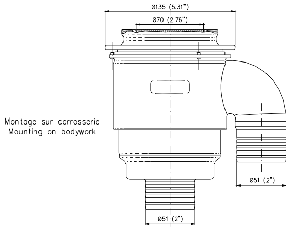
Accoupleur femelle
