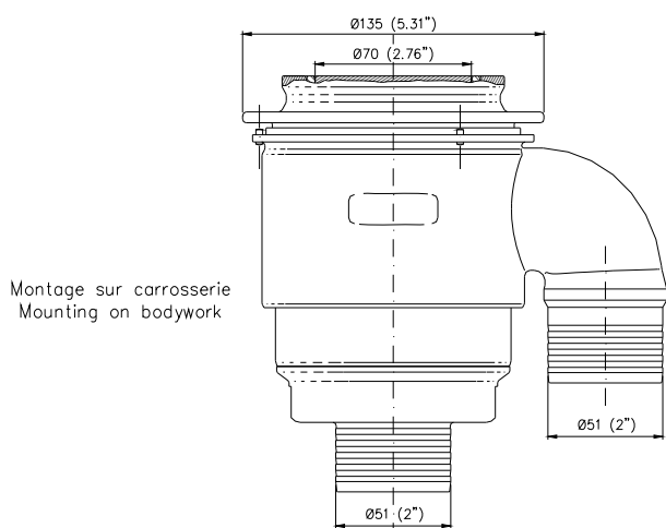
Accoupleur femelle
